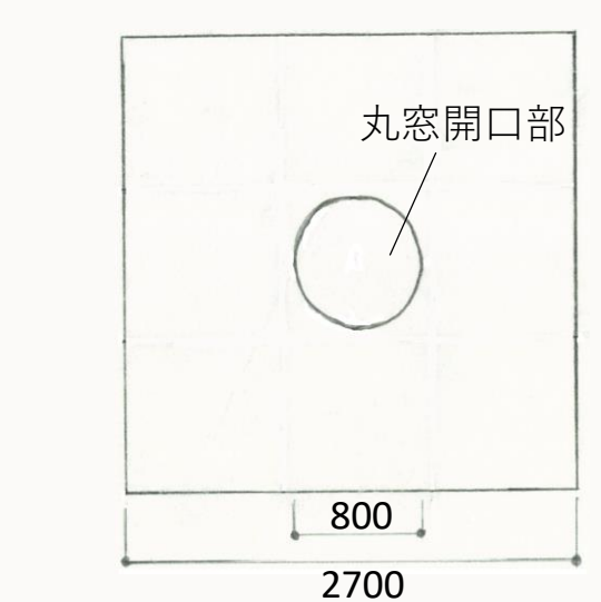
展開図（東） 1/50
