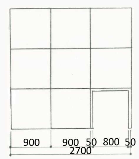
立面図（西） 1/50
