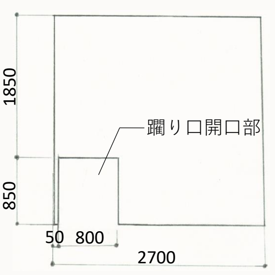
展開図（西） 1/50
