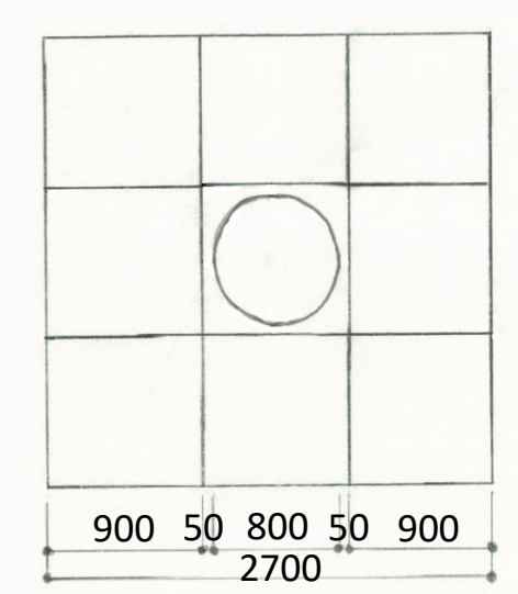
立面図（東） 1/50
