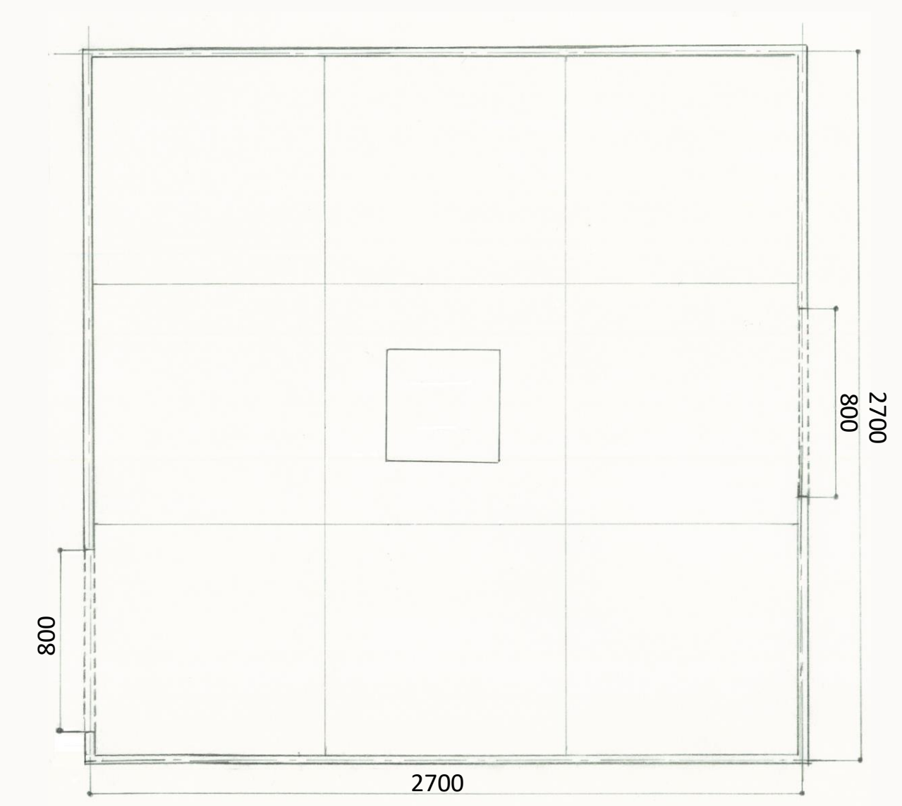
平面図 1/20
